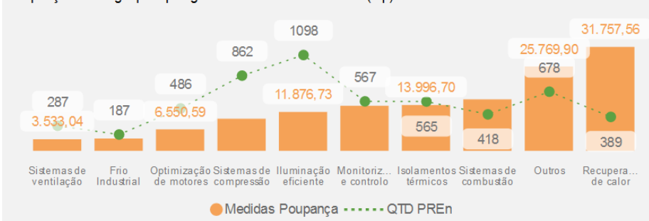
Economia, investimento e PRI médio por tipologia de submedida transversal
