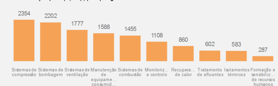
Custo de redução por tep (€/tep) por tipologia de submedida transversal
